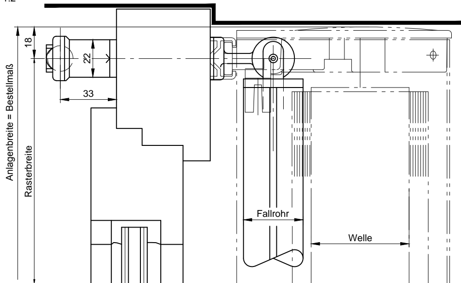
Horizontalschnitt M 1:2
