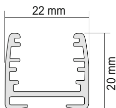
Profilo maxi
