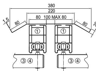
Abdeckblech Doppelführung
