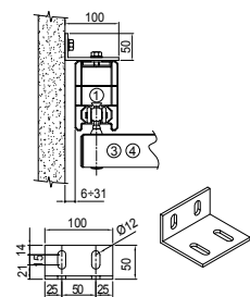
*Befestigungswinkel
