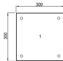
Abmessung Fussplatte
