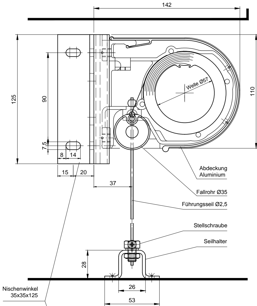
Vertikalschnitt M 1:2
